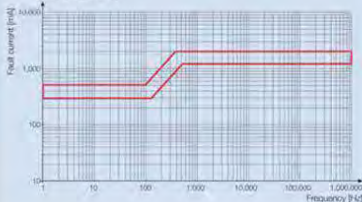
RA4xxx 500 mA
