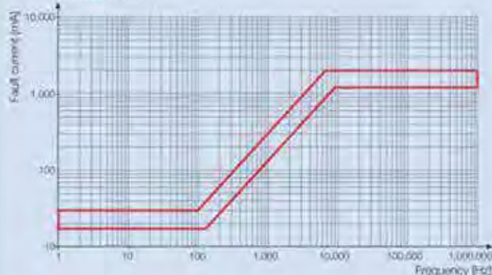
RA4xxx 30 mA
