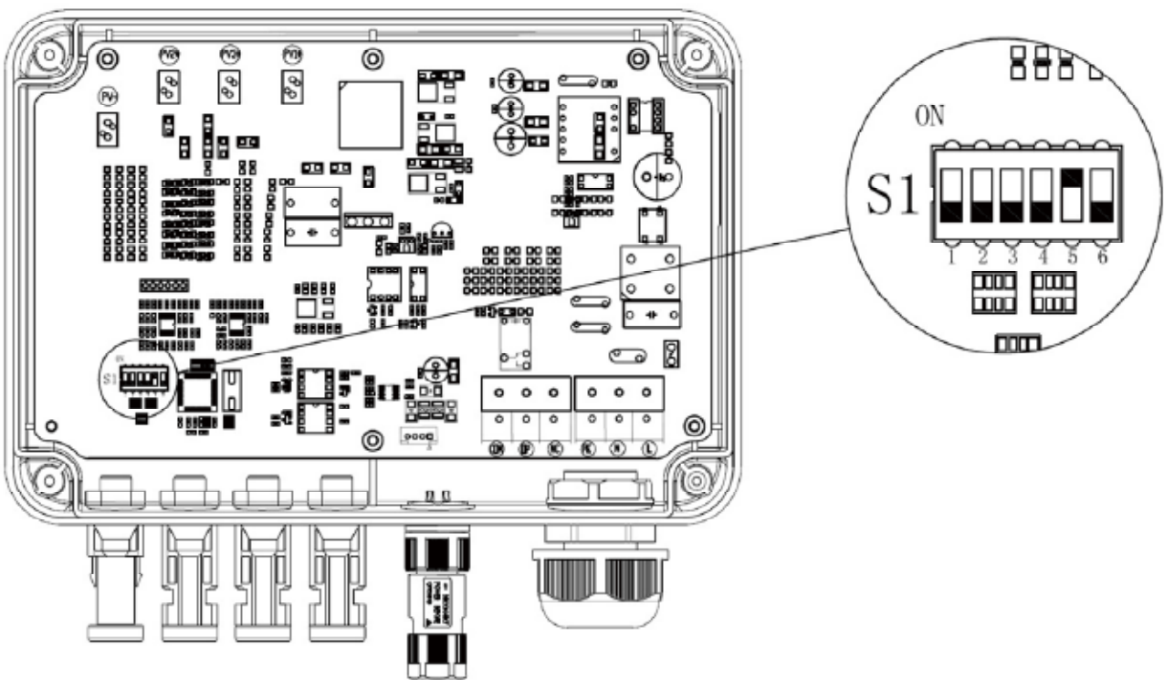
6 位元撥碼開關位置示意图
