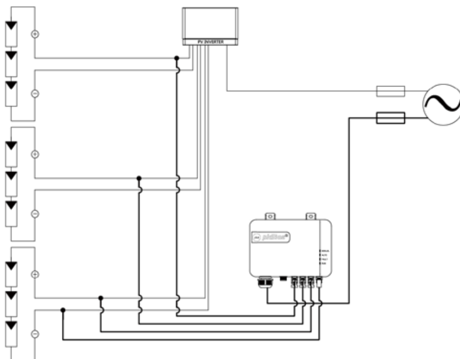
3路 MPPT 連接示意圖
