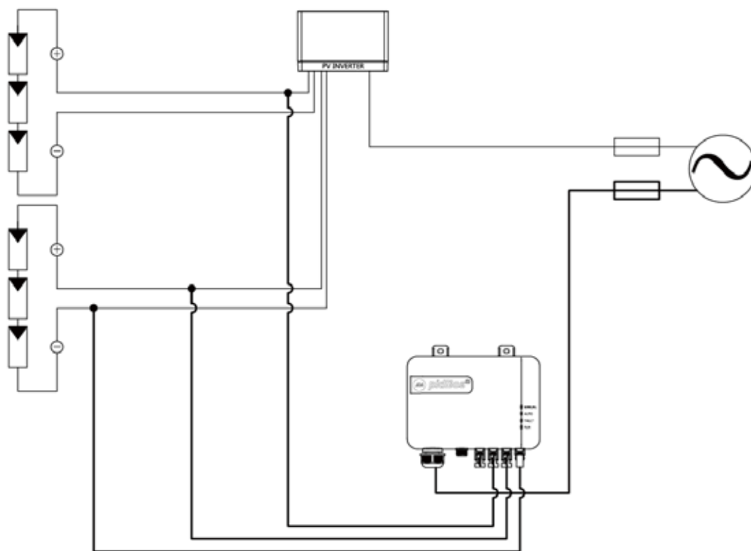
2路 MPPT 連接示意圖
