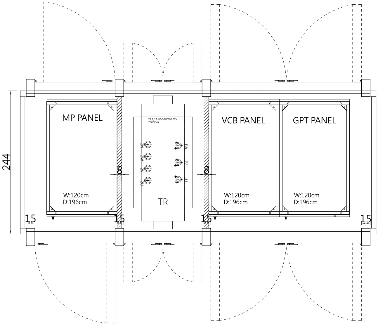
配置俯視圖
