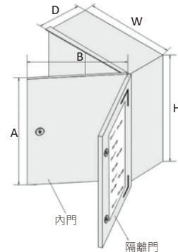
玻璃纖維強化塑膠箱 ( 玻璃纖維箱 · GRP 箱 )
