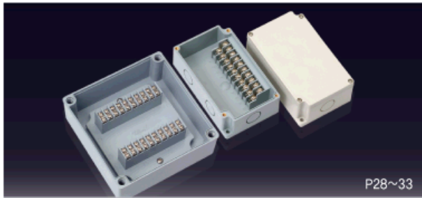
단자박스 - Terminal Block Box
